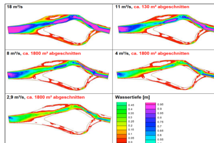
Modélisation 2D CASIMIR
